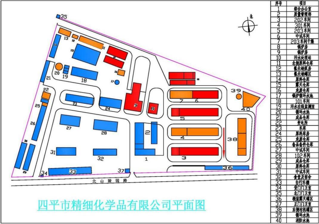
图 4-1 厂区平面布置图
